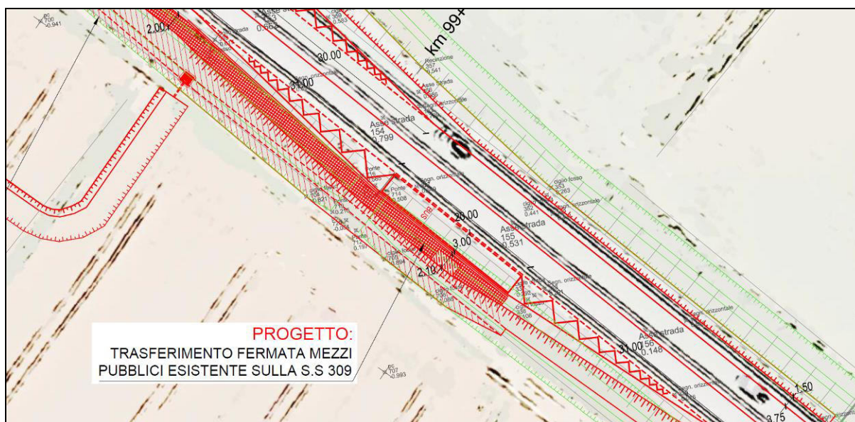
Figura 20 – Stralcio planimetrico della fermata in direzione Chioggia
